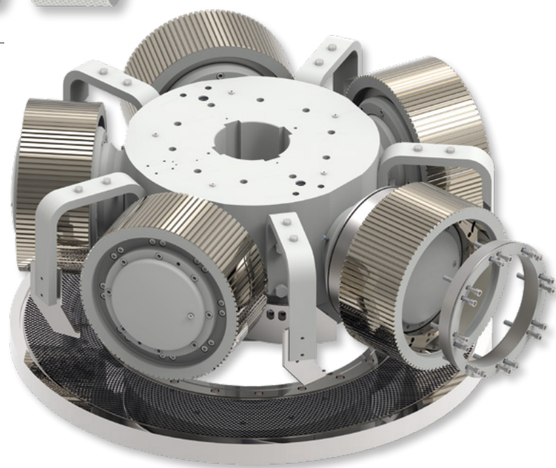
↑ Tête de galets sur la filière plate
